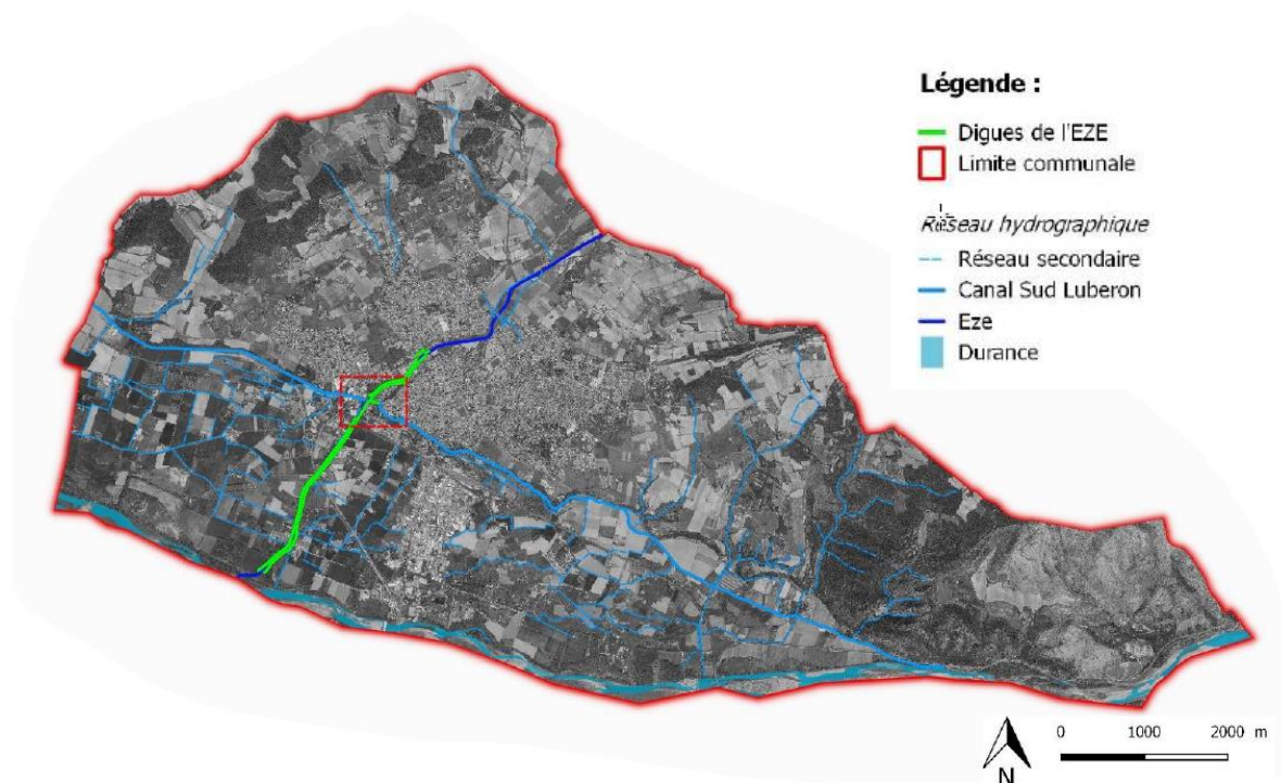
L'Eze à Pertuis (source : Diagnostic initial des digues de l'Eze – SCE)
