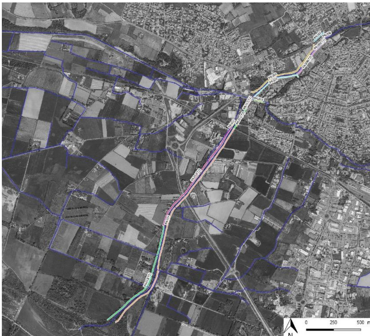
Ouvrages concernés par la présente convention (source : Diagnostic initial des digues de l'Eze – SCE)
