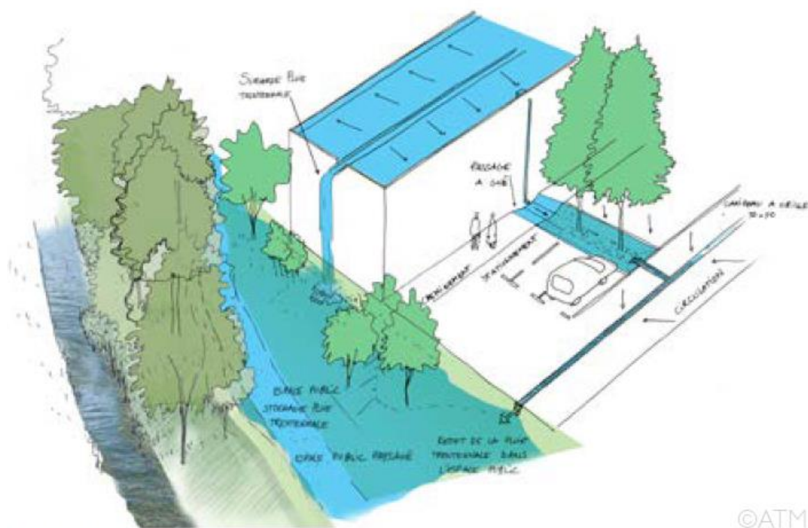
Figure 11 : Exemple lot 5 lors d'une pluie trentennale
