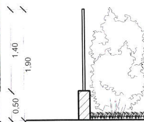
Maçonnerie enduite, grille métallique peinte, haie vive
