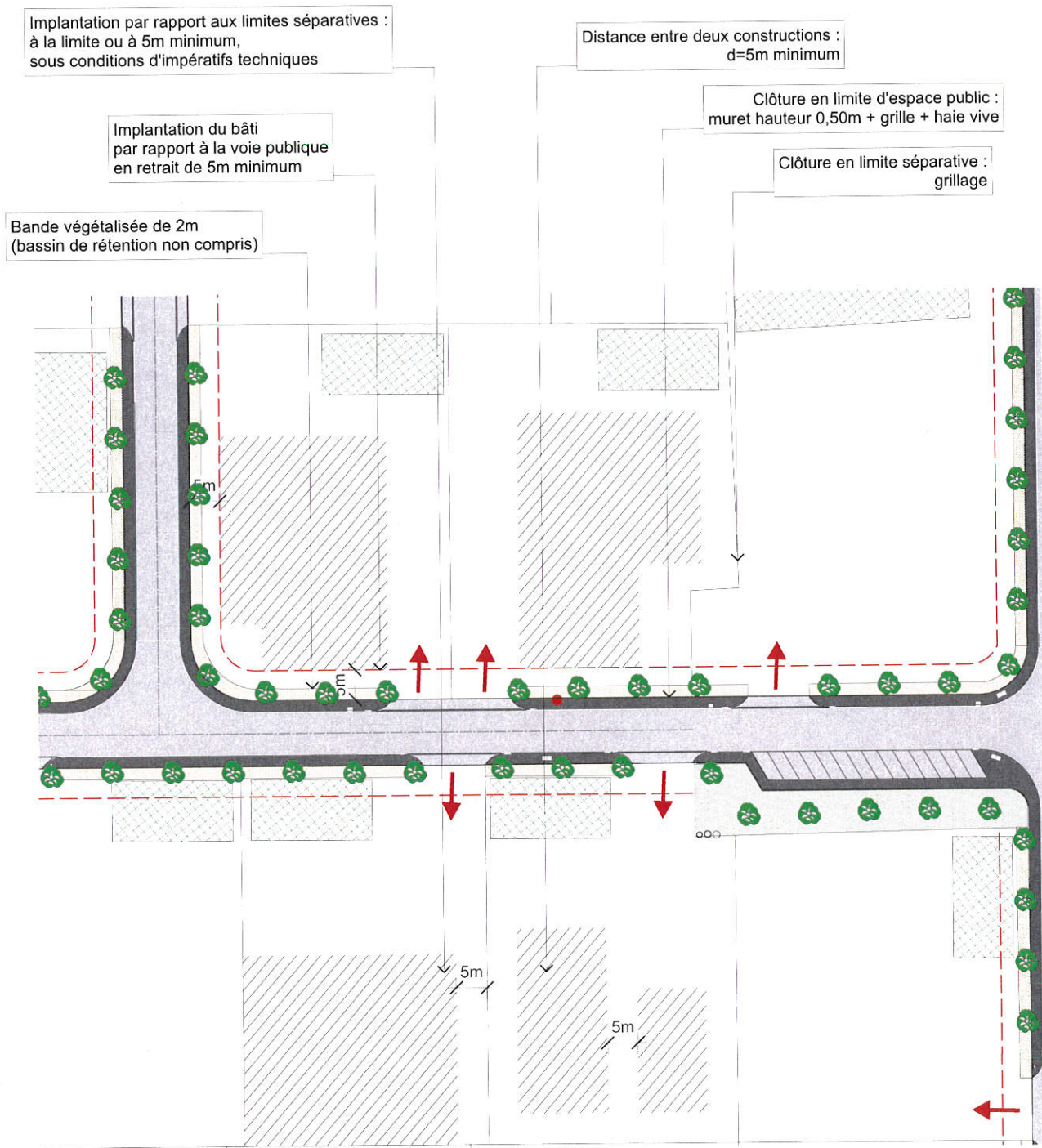
SCHÉMA D'IMPLANTATIONS POSSIBLES
