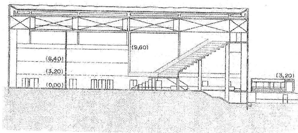
Coupe longitudinale de la Salle
