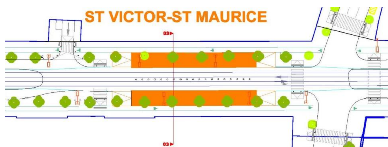
Figure 18 : Station Saint-Victor - Saint-Maurice - Variante d'insertion latérale (variante privilégiée)
